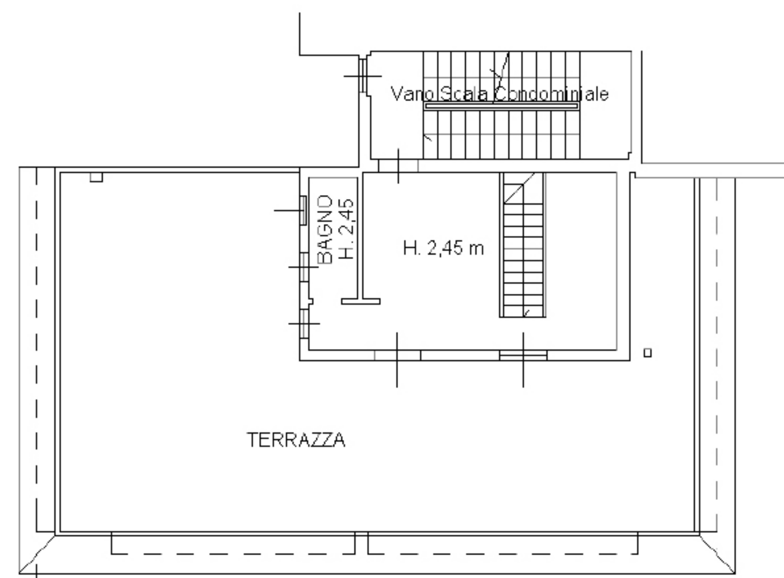
PIANO SECONDO
