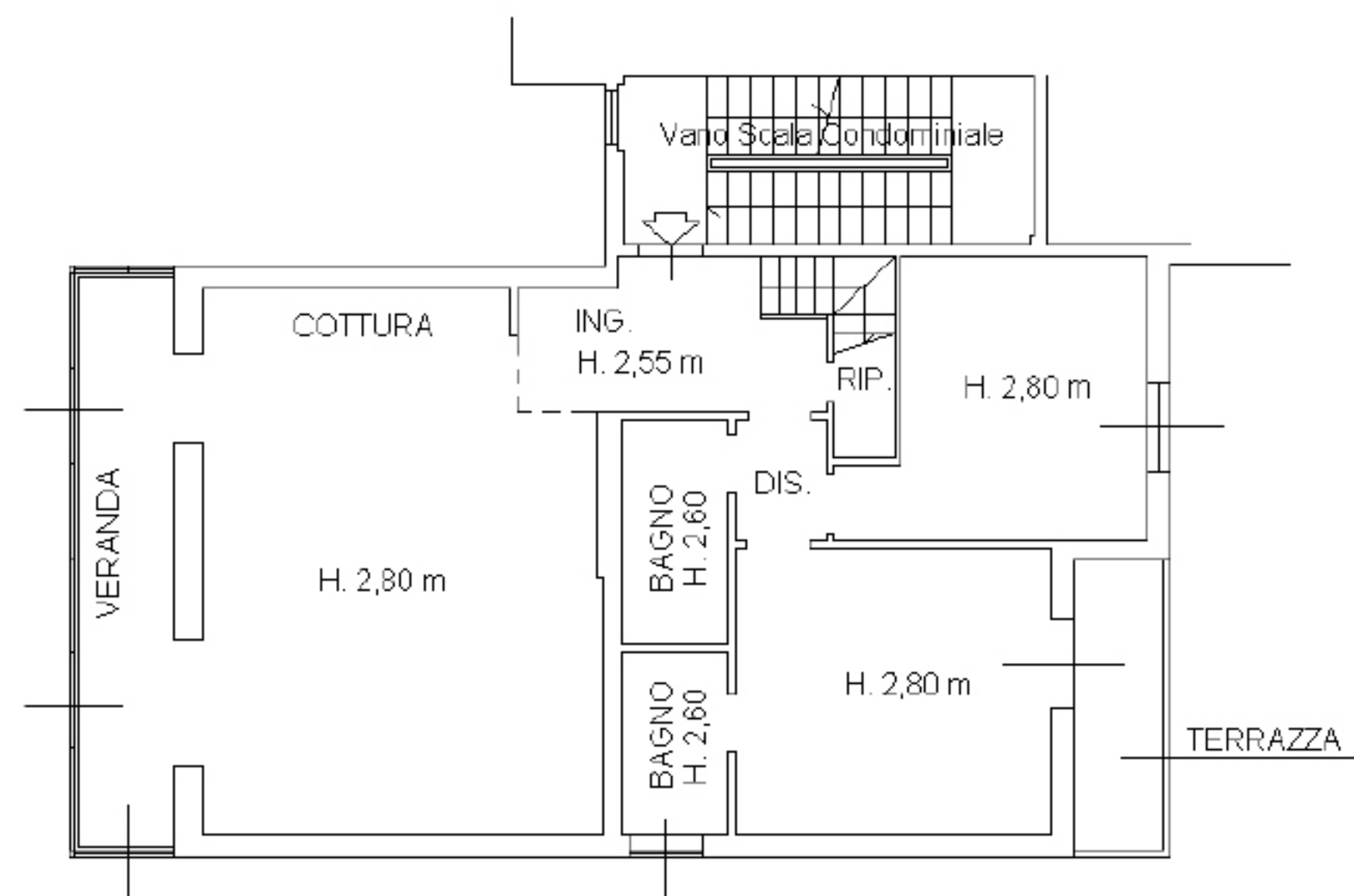
PIANO PRIMO
