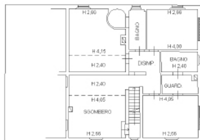
PIANO PRIMO
